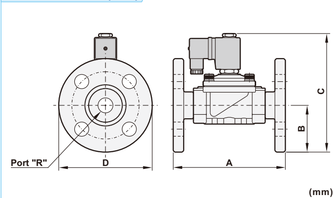
SPU220A 法蘭型(10K)
