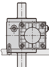
底座固定
