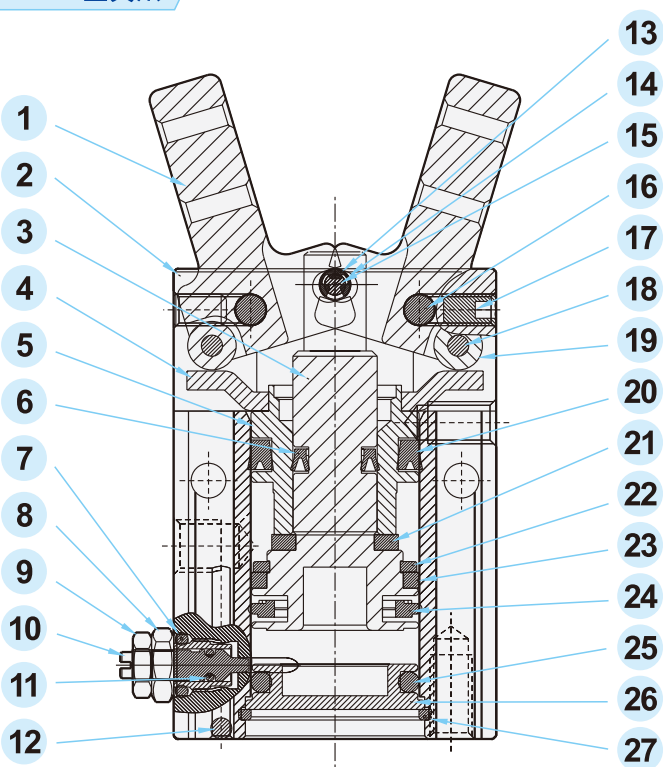
HYS：Y型夾爪
