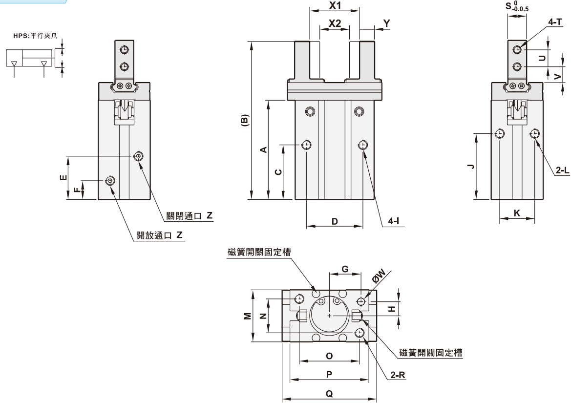
HPS-10~25
